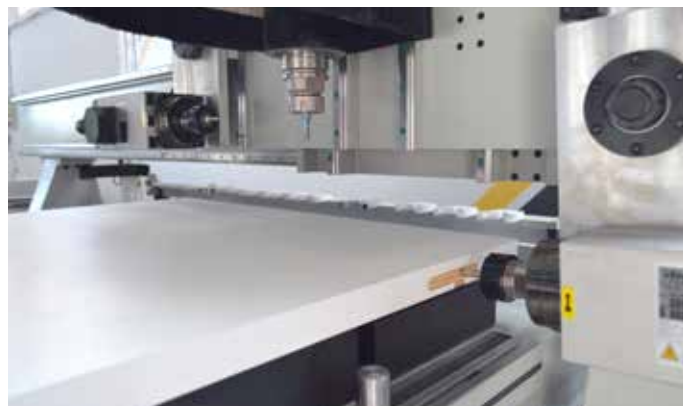
Detalle grupo de trabajo, cambio lineal, ventosas. Mecanizado de pernio.
